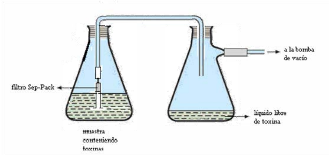
Fig. 11. Equipo para concentración de toxinas contenidas en muestras de agua de red
