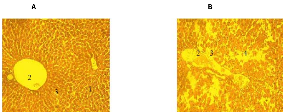
Fig. 2: Corte de hígado de ratón control (A) de un ratón inyectado con extracto acuoso de Microcystis sp. obtenida de un florecimiento natural de río de la Plata (B). 1- Vena hepática terminal 2- Tracto portal 3- Interface del parénquima en posición radiada. Nótese tracto portal con importante vasodilatación, disrupción de la interfase del parénquima y pérdida parénquima hepático.
