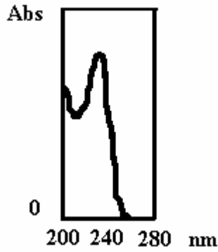
Fig. 18. Espectro de absorción UV de MCs
