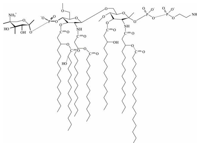
Fig. 10. Estructura de Lipido A, El componente tóxico de los LPS
