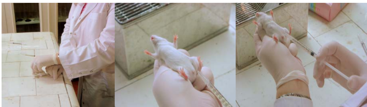
Fig. 12. Técnica de inmovilización e inyección de un ratón
