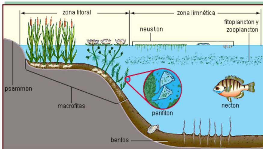
Fig. 1. Esquema de un cuerpo de agua donde se señalan las diferentes comunidades
