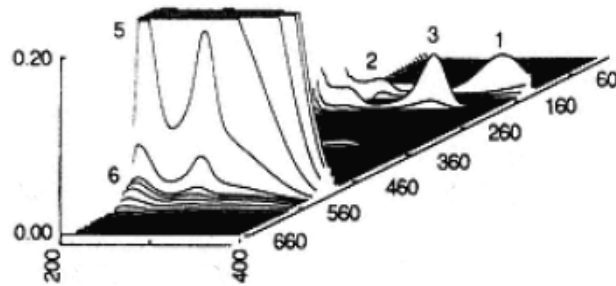
Fig. 6: Cromatograma en representación tridimensional mostrando el espectro entre 200 y 400 nm de cada pico eluido.
