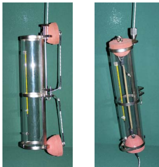
Fig. 4. Botella de Van Dorn abierta y cerrada
