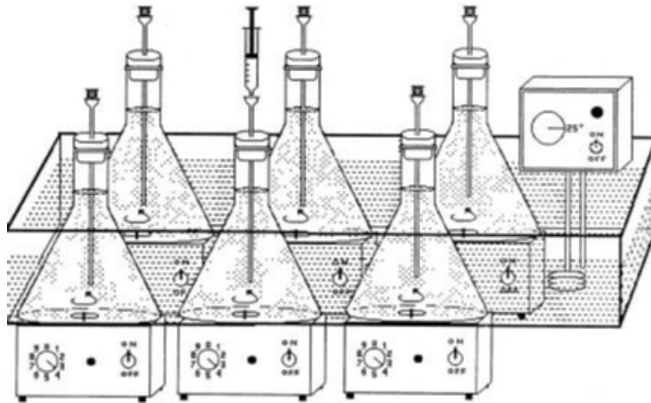
Fig. 4: Reactores para ensayos con carbón
