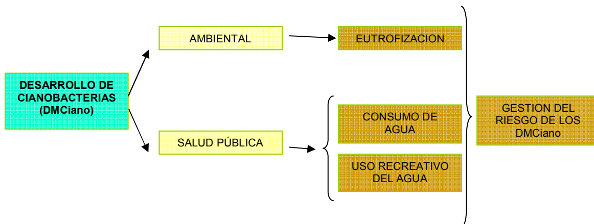
Fig. 1: Esquema de la problemática causada por el desarrollo masivo de Cianobacterias (DM Ciano)
