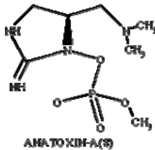
Fig. 9: Estructura de la anatoxina-a(s)
