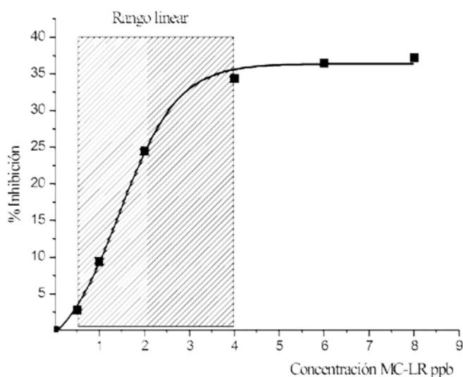
Fig. 14. Curva de calibración % Inhibición vs. Concentración MC-LR para el ensayo de inhibición de proteína fosfatasa. El área rayada indica el rango lineal del método.
